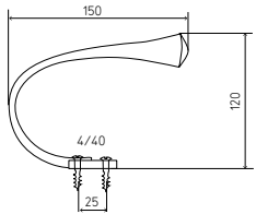
EMBRASSE FIXE
